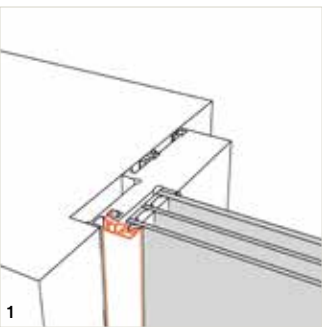
ingombro minimo dei profili
