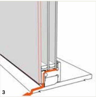
zoccolatura rivestita di vetro, scarico acqua nascosto
