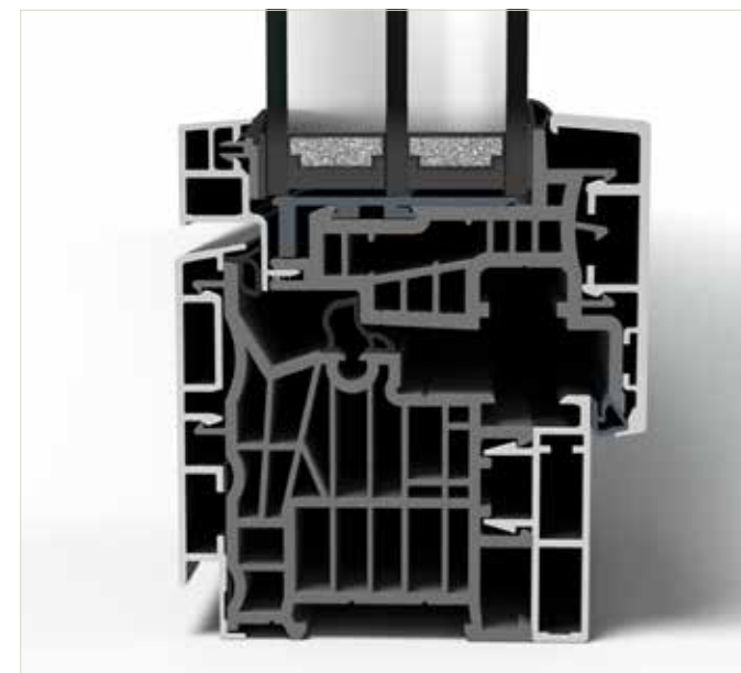
Sezione di un profilo in alluminio Finstral: FIN-Project Slim-line 78 alluminio-alluminio
