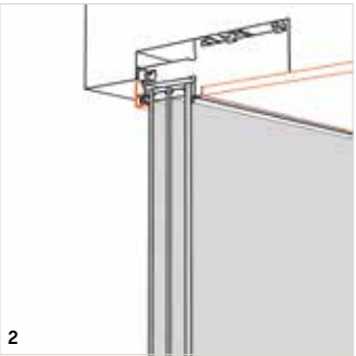
interno: montaggio a scomparsa
